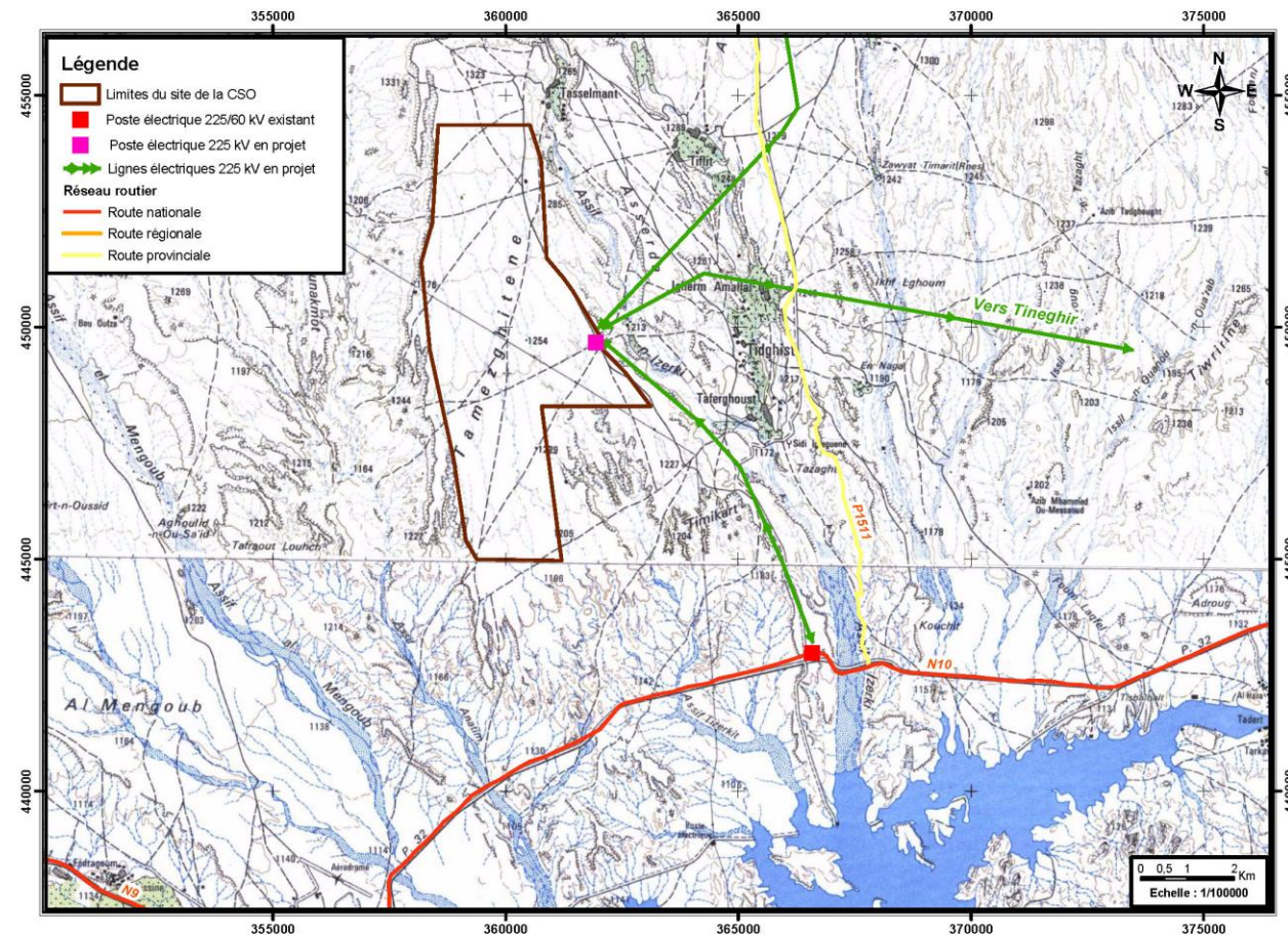
Figure 23 : Localisation du futur poste ONE 225kV au niveau du site et projection du couloir de la ligne de rabatement
